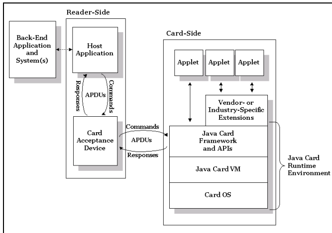
Gambar 9 Arsitektur Aplikasi Java Card
