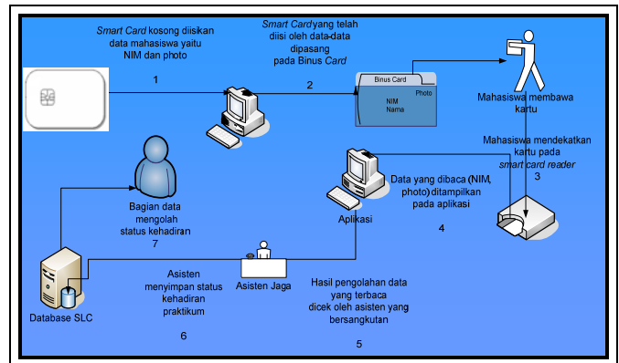
Gambar 11 Model Konseptual Proses Pengisian Kehadiran Praktikum dengan Smart Card
